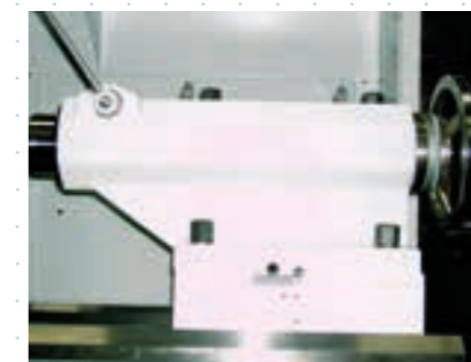
Verstärkter Reitstock mit Pinolendurchmesser 140 mm (nur bei E80)
