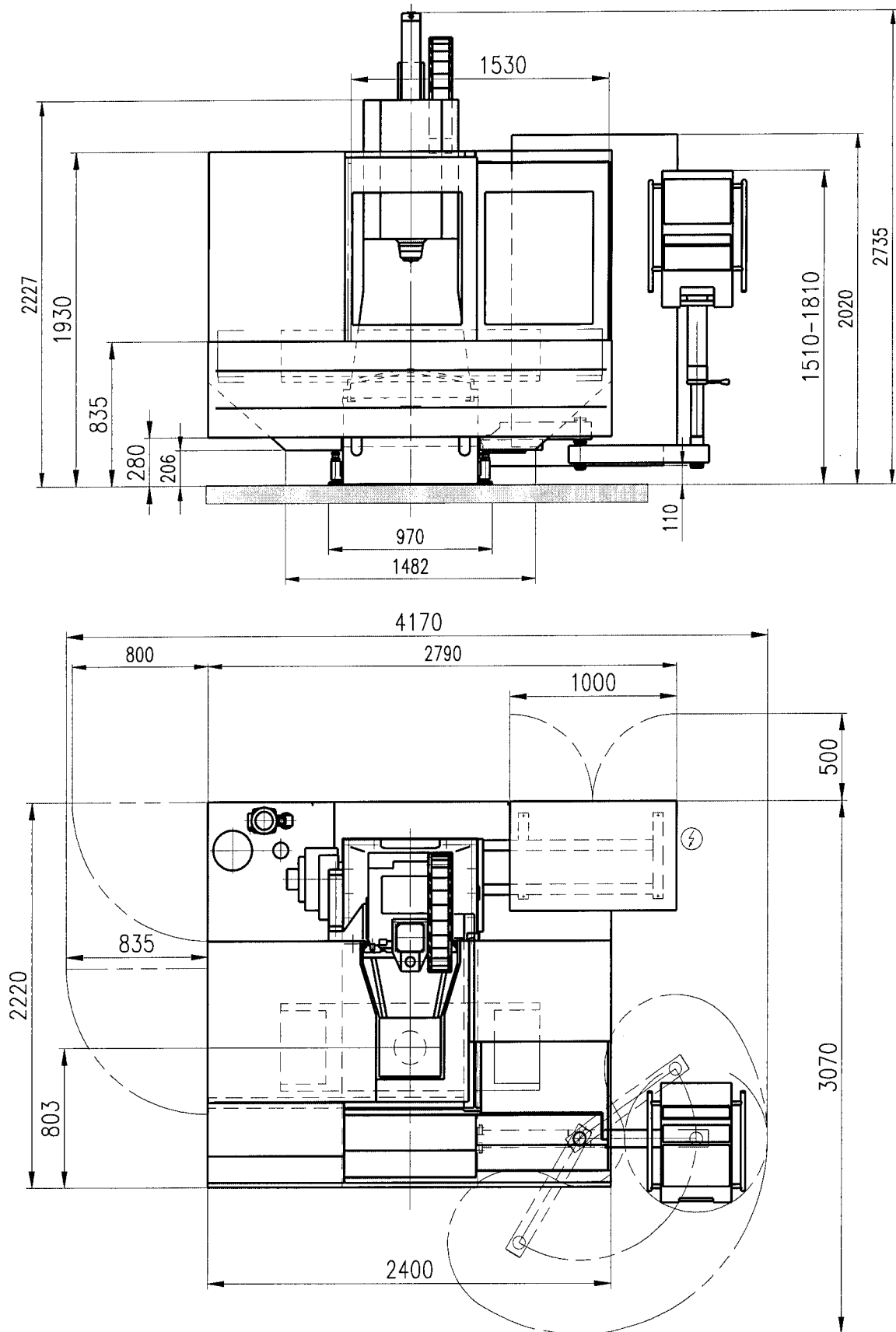
Abbildung 22: Maschinen-Maßbild
